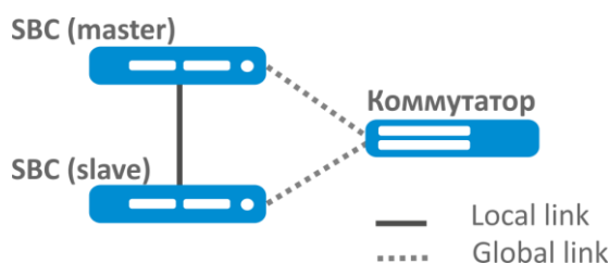
Рисунок 2 – Резервирование Eltex SBC по схеме active-backup
