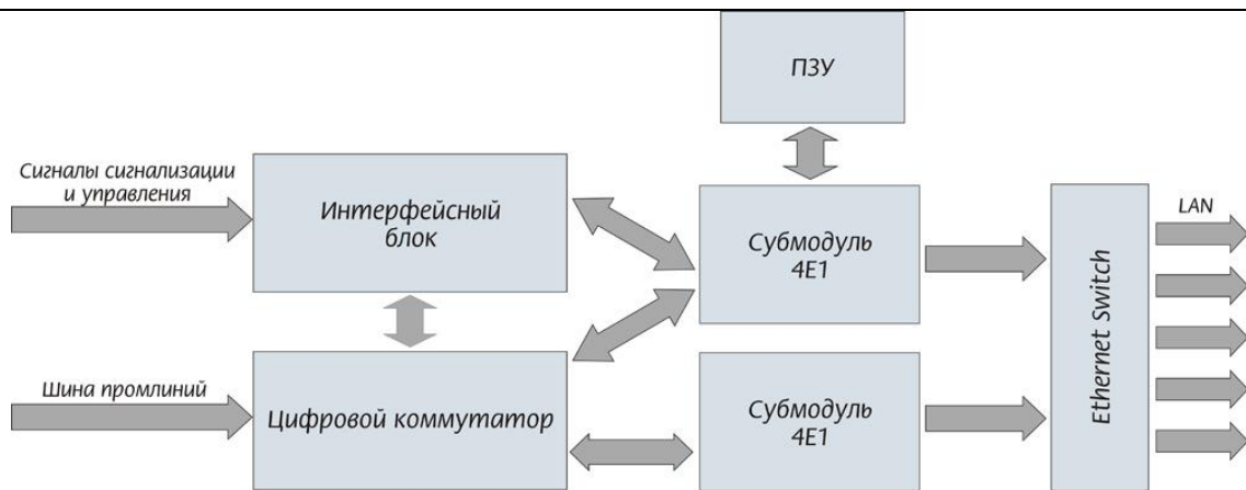
Рисунок 6 – Функциональная схема модуля TM.IP
