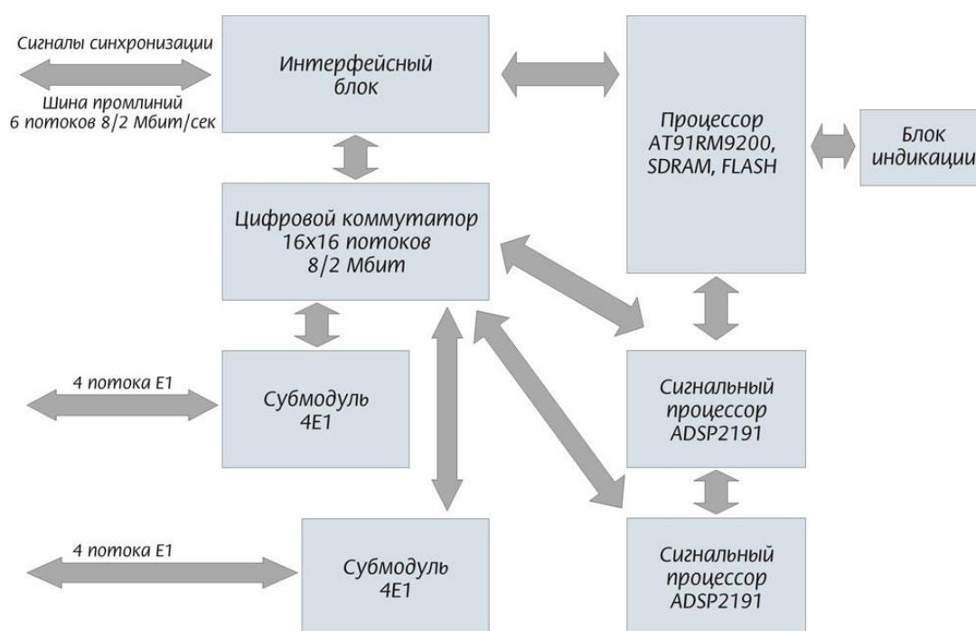
Рисунок 5 – Функциональная схема модуля 8ТМ
