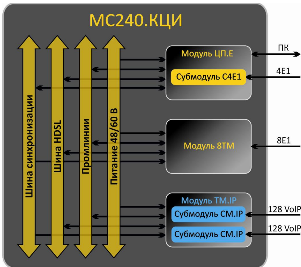
Рисунок 1 – Архитектура конвертора цифровых интерфейсов «MC240»
